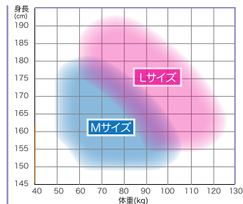
フルハーネスサイズ表
